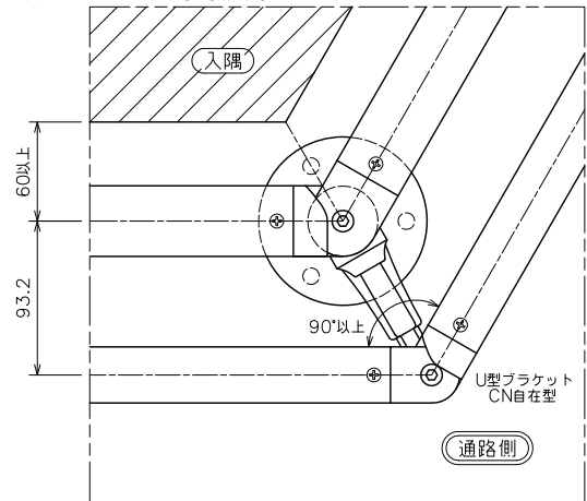
< 外コーナー 90度以上 >
