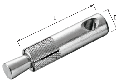
石引アンカー
