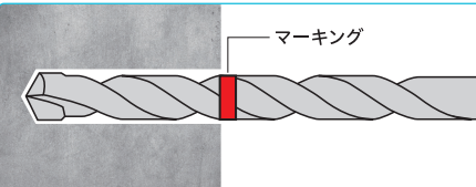
【石引アンカーの施工方法】
