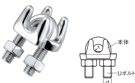
ワイヤークリップ
