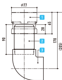
消雪用ドレン〈50型セット〉
