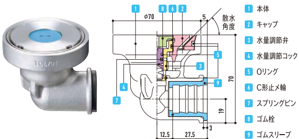
● 寸法図
