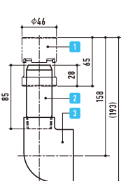
消雪用ドレン〈25型セット〉
