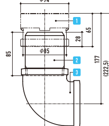
消雪用ドレン〈65型セット〉
