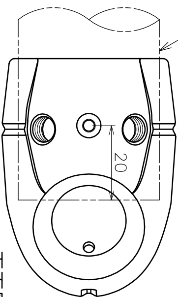
下面図
