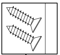
注5) 十字穴付皿タップピンねじ φ4.1×16 2個 SUS304
