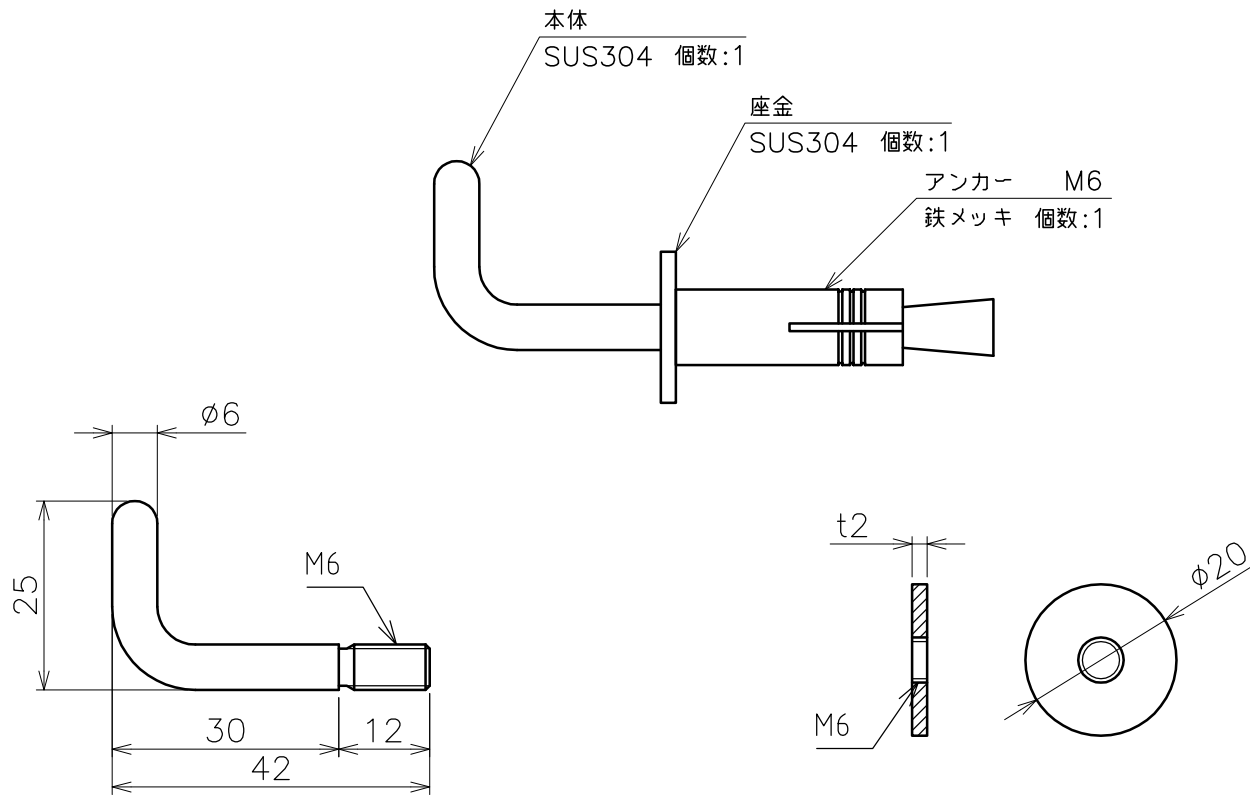
本体詳細
