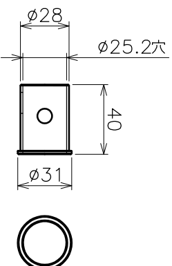
⑤ A部スリーブ詳細図 (S=1:2)
