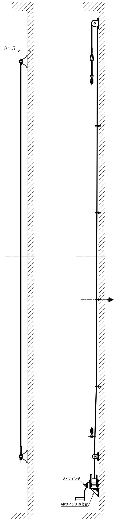
サイドワイヤー部 吊ワイヤー部
