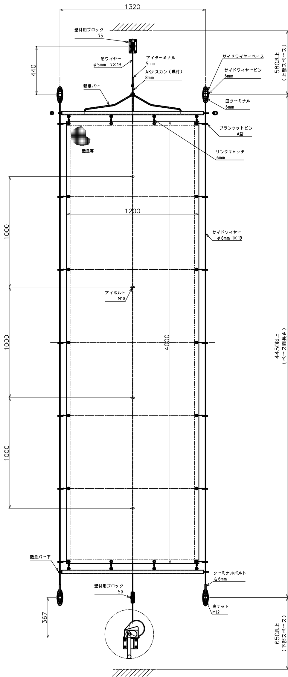
サイドワイヤー部 吊ワイヤー部
