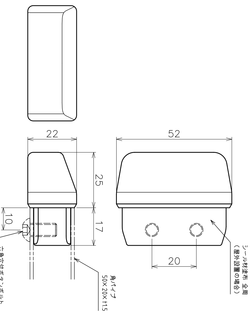
<Kエントキャップ詳細>
