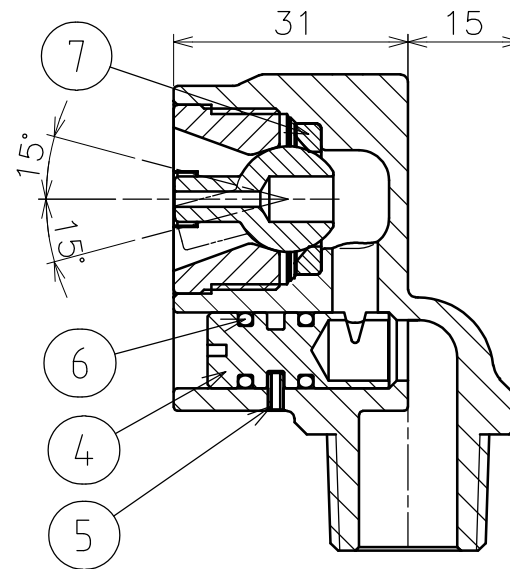
A-A断面
