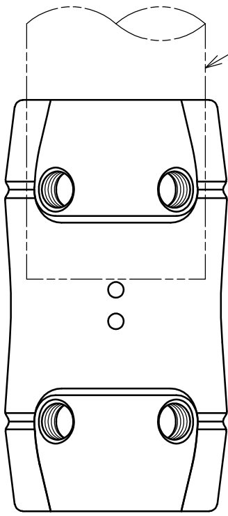
下面図
