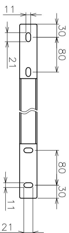
平面/下面図 アンカー長穴詳細 (S=1:5)
