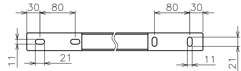
平面/下面図 アンカー長穴詳細 (S=1:5)
