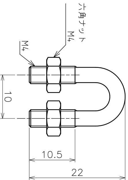
Uボルト
