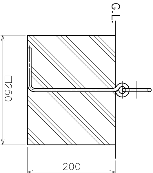
施工参考図 (S=1:5)
