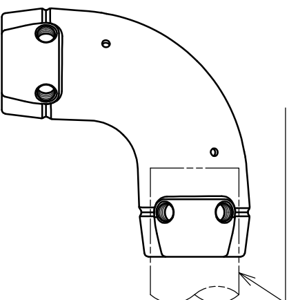
矢視図 (S=1:2)
