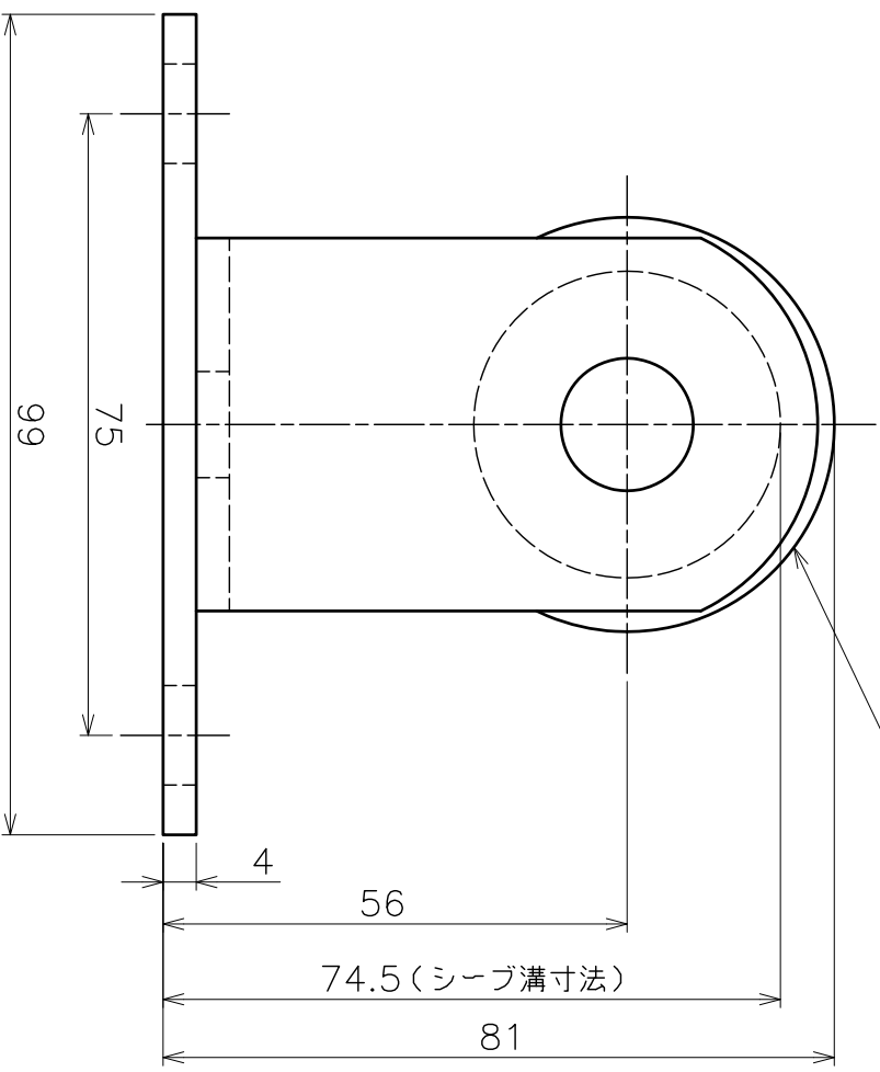
ASANO溶接用ブローク (サイズ50, AK10040)
