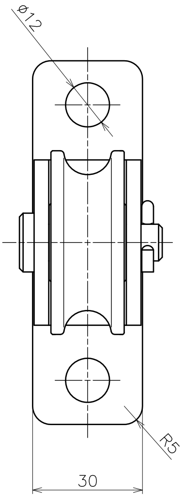
ASANO溶接用ブローク (サイズ50, AK10040)
